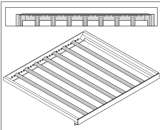
Fig. 90 Розташування планок для максимальної кількості пляшок.
